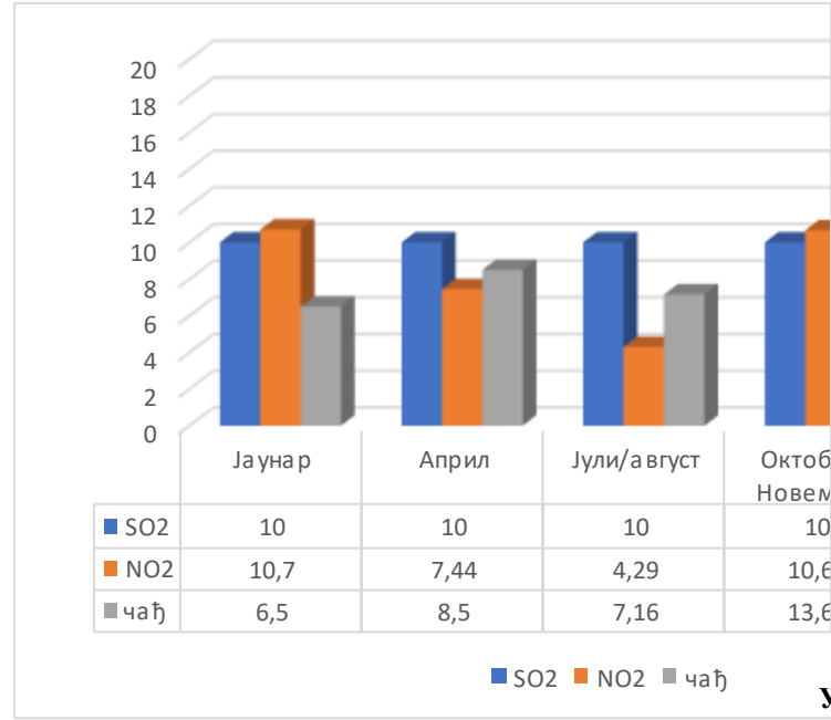
Упоредни преглед средње концентрације: SO 2 , чађи и NO 2 .
